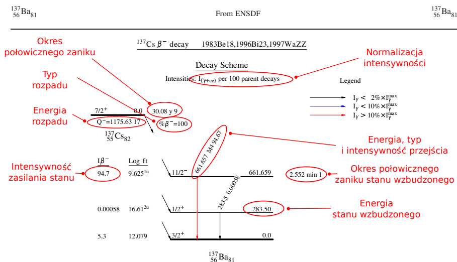
Rysunek 5: Schemat rozpadu ^{137}\text{Cs} [9].
