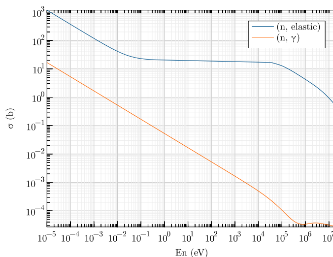
Rysunek 7: Zależność przekroju czynnego dla wodoru ( ^1\text{H} ) na rozproszenie elastyczne ( n + p \rightarrow n + p ), oraz na wychwyt neutronu ( n + p \rightarrow d + \gamma ).
