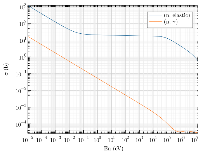
Rysunek 9: Zależność przekroju czynnego dla wodoru ( ^1\text{H} ) na rozproszenie elastyczne ( n + p \rightarrow n + p ), oraz na wychwyt neutronu ( n + p \rightarrow d + \gamma ).
