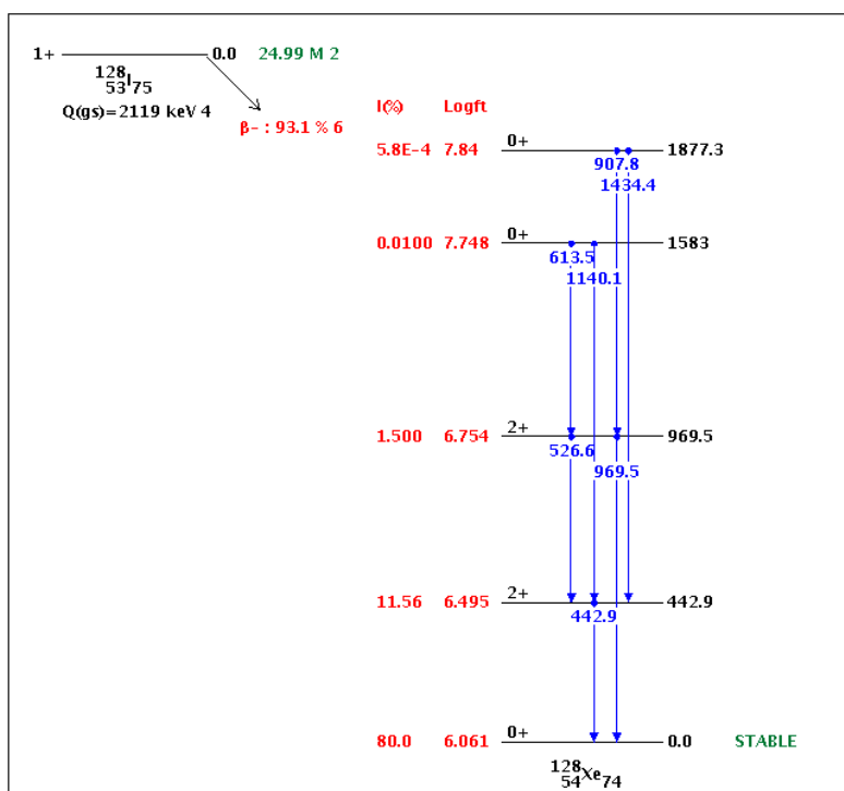
Rysunek 2: Schemat rozpadu ^{128}\text{I} na drodze przemiany \beta^- .
