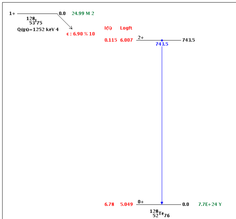
Rysunek 3: Schemat rozpadu ^{128}\text{I} na drodze wychwytu elektronu.
