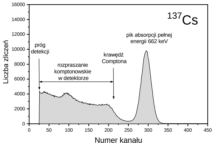
Rysunek 5: Przykładowe widmo promieniowania \gamma zarejestrowane przez detektor scyntylacyjny NaI(Tl) dla źródła ^{137}\text{Cs} .
