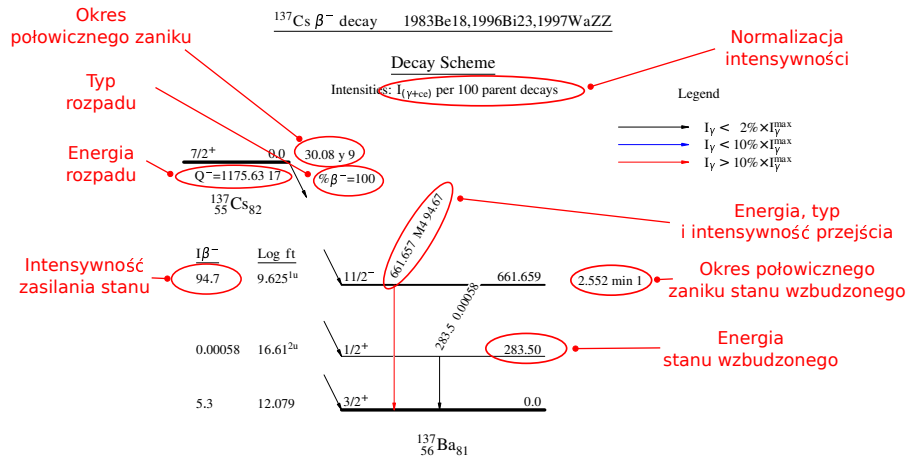
Rysunek 7: Schemat rozpadu ^{137}\text{Cs} [?].
