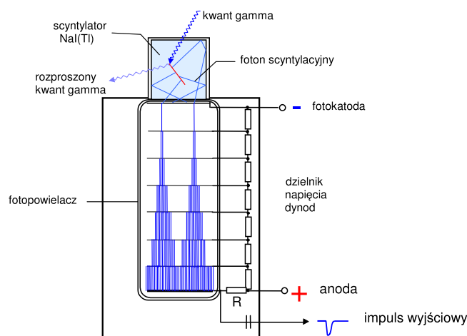
Rysunek 6: Schemat budowy detektora scyntylacyjnego.
